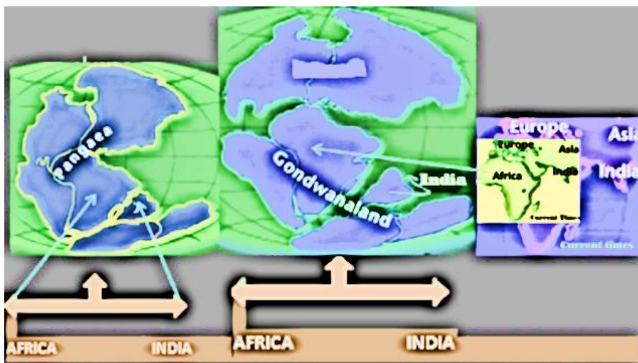
fig. Pangaea&gt;LG&gt;Hexarchy
