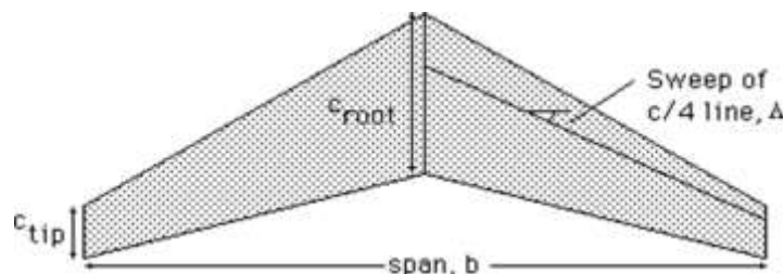
Fig 1: Wing Design Parameter
